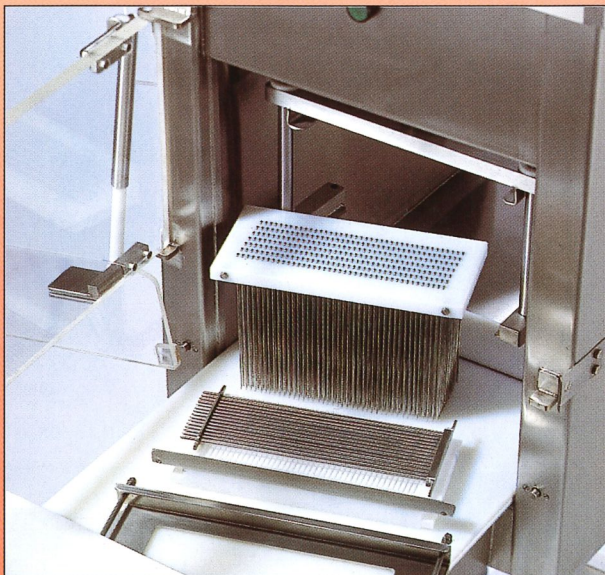
Bloc-lames démontable.
