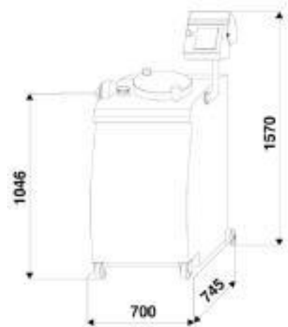
Abmessungen Torsado
